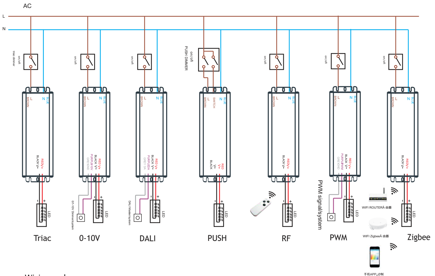
Wiring color
